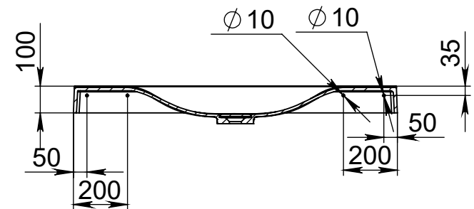
B-B
